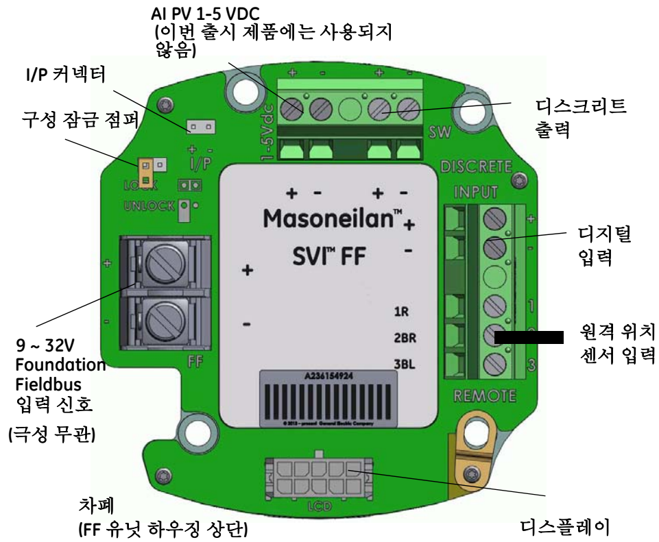
그림 1 전자 장치 모듈 측 연결부(단자반을 통해)
